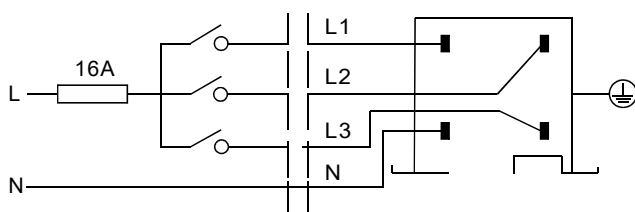
1 Phase / 单相电 230VAC 16A Max
